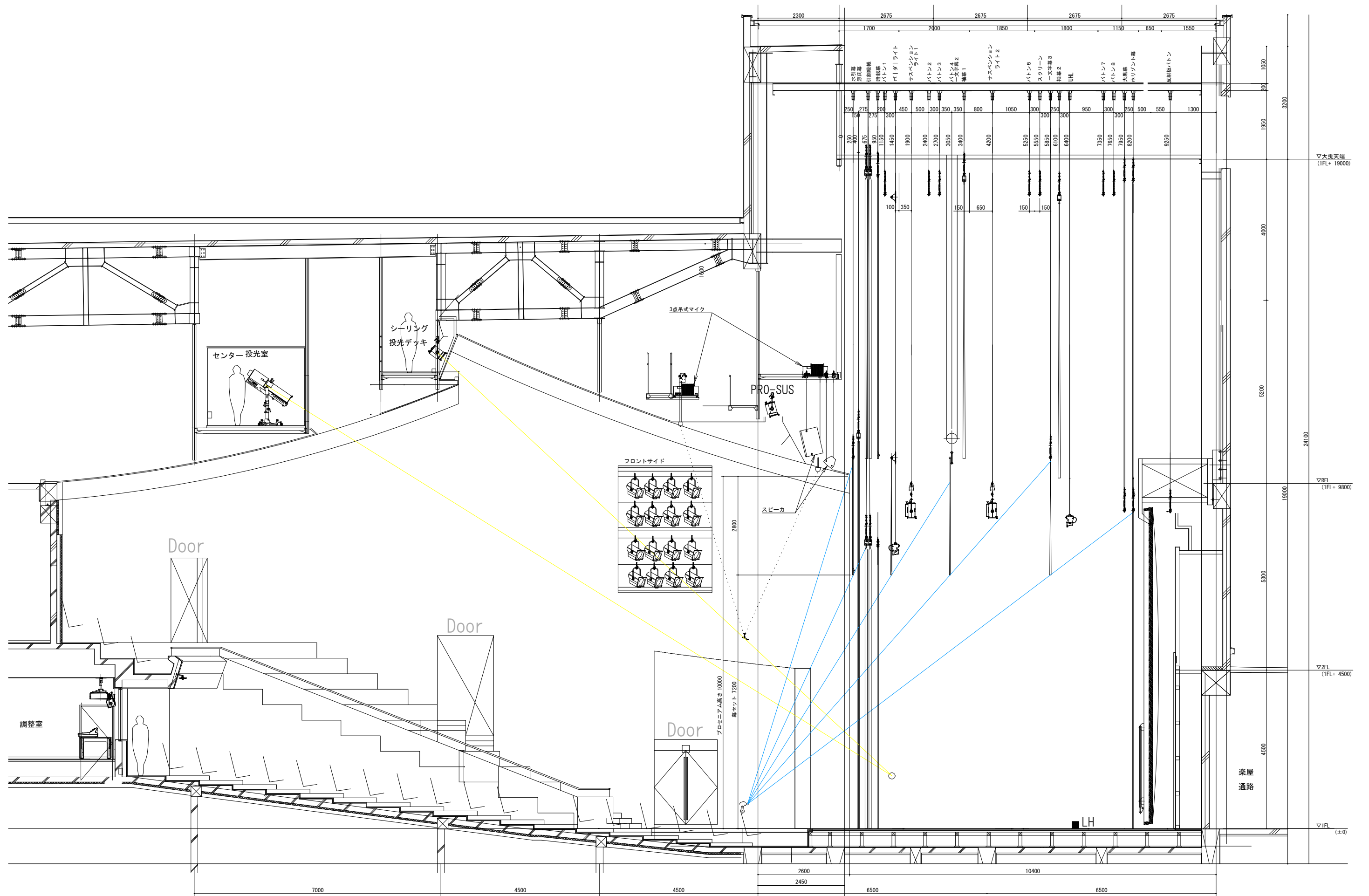
藍住町総合文化ホール 舞台機構設備 断面図
